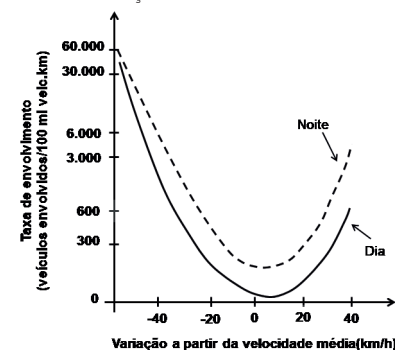
Figura 3.1 - Taxa de envolvimento em sinistros em função da variação da velocidade média
