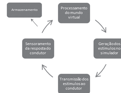
Figura 14.1 – Componentes de um simulador de direção.
