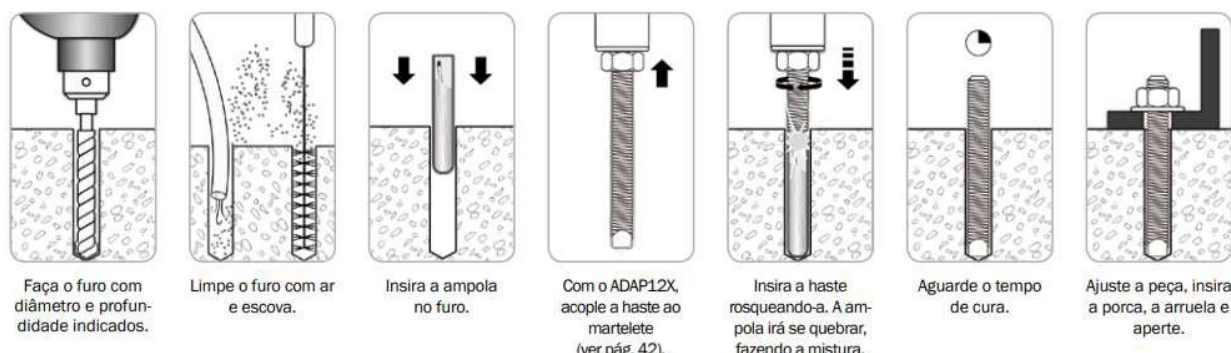
Figura 1 – Método de aplicação da ancoragem química AQA Epóxiacrilato (Fonte: Catálogo Técnico Âncora 2019)
