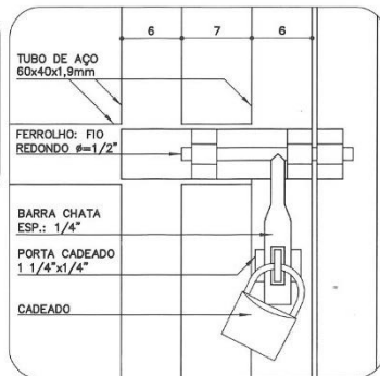
DETALHE 4A ESC. 1:5
