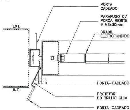
DET. PROTETOR DO TRILHO-GUIA (POSIÇÃO PORTÃO FECHADO) ESC. 1:5
