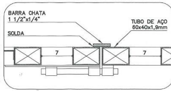
DETALHE 2A ESC. 1:5
