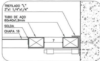
DETALHE 2A ESC. 1:5
