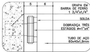
DETALHE 3 ESC. 1:5
