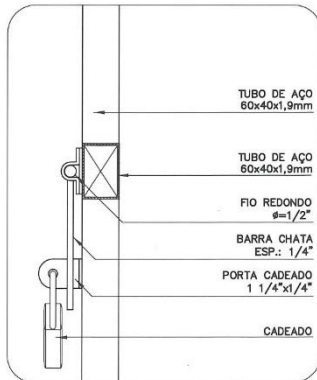
DETALHE 4A E 4B VISTA LATERAL ESC. 1:5
