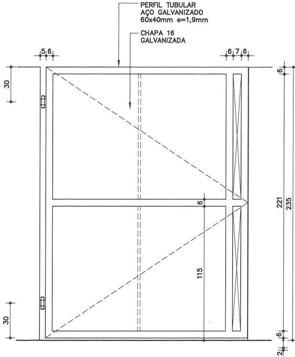
VISTA EXTERNA PT-42 ESC. 1:25
