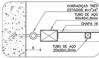
DETALHE 1 ESC. 1:5
