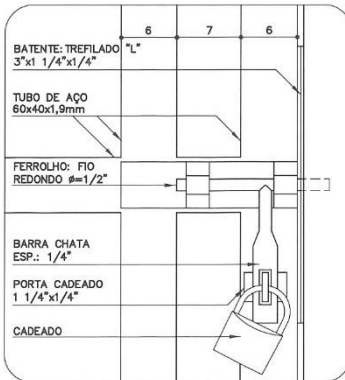
DETALHE 4B ESC. 1:5
