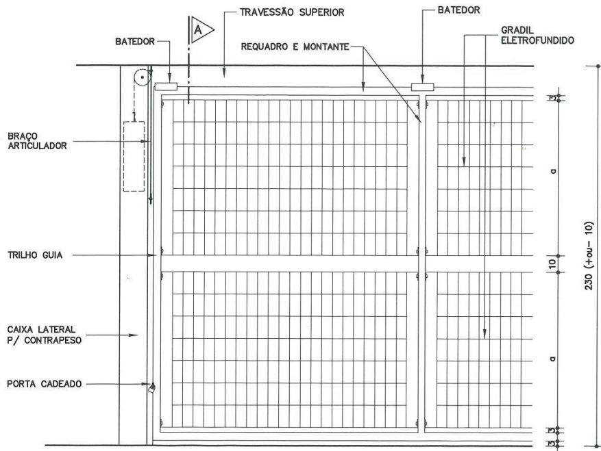
AMPLIAÇÃO PARCIAL – VISTA INTERNA ESC. 1:25
