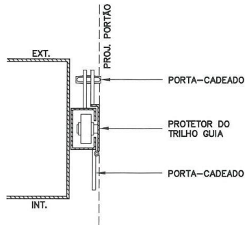
DET. PROTETOR DO TRILHO-GUIA (POSIÇÃO PORTÃO ABERTO) ESC. 1:5
